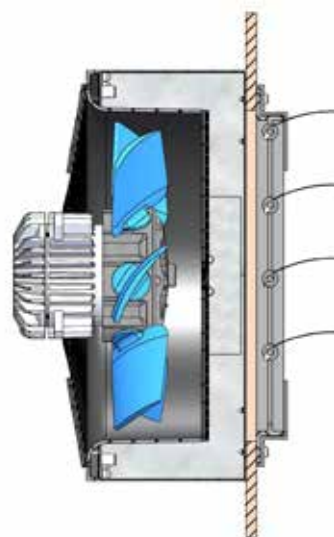
INSTALLAZIONE A PARETE CON DISTANZIALE WALL INSTALLATION WITH MOUNTING SPACER
