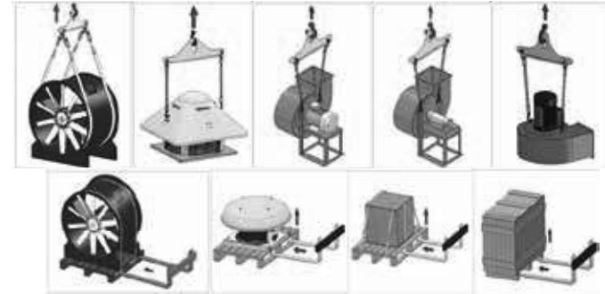
FIG.1 –TRASPORTO E INSTALLAZIONE / TRANSPORT AND INSTALLATION
