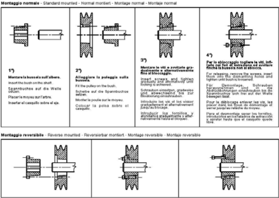
Fig. 3 –SMONTAGGIO E MONTAGGIO PULEGGE / DISASSEMBLY AND ASSEMBLY PULLEYS
