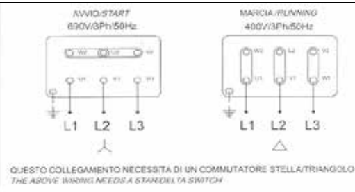
FIG. 1 –SCHEMI DI COLLEGAMENTO ELETTRICO PIU' COMUNI / MOST COMMON WIRING DIAGRAMS
