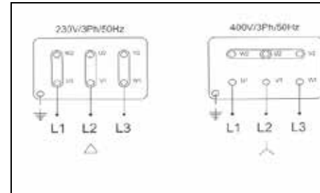
FIG. 1 –SCHEMI DI COLLEGAMENTO ELETTRICO PIU' COMUNI / MOST COMMON WIRING DIAGRAMS
